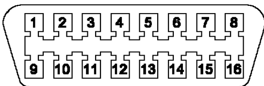
Pinbelegung des Diagnosesteckers am Fahrzeug, Vorderansicht
