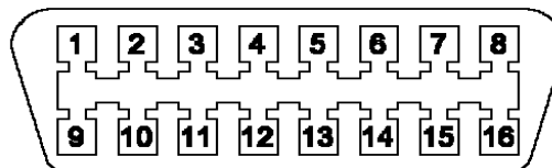
Vorderansicht, Pinbelegung OBD2
